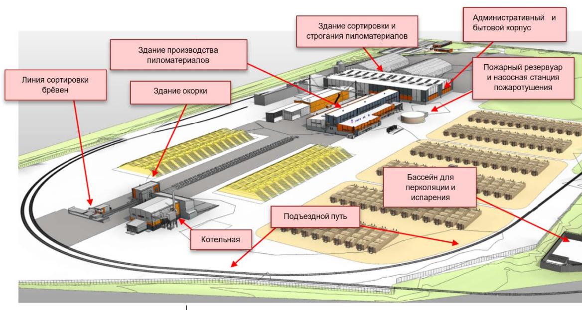
Рисунок 2-4 – Схематический план расположения объекта
